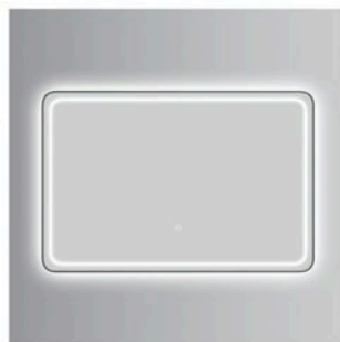
KR604L 尺寸Size: 800x600/700x500mm 输入电压: AC110-240V 50/60Hz 输出电压: DC12V 输出电流: 1A/2A/3A 额定功率: 12W/24W/36W 镜子功能: 触控灯光 材质: 太空铝斜边框
